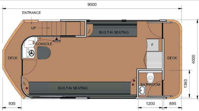
Floor Plan N.T.S.
